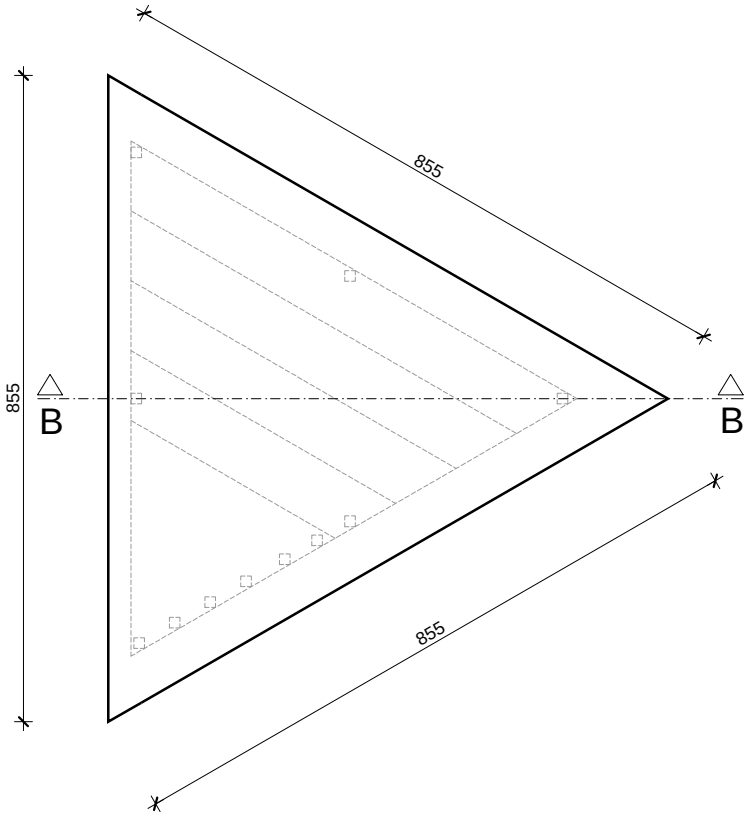
Krovne plohe
