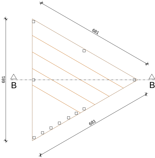
Tlocrt prizemlja
